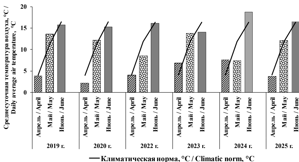
Рис. 2. Среднесуточная температура воздуха весенне-летнего вегетационного периода / Fig. 2. Daily average air temperature of the spring-summer vegetation period
