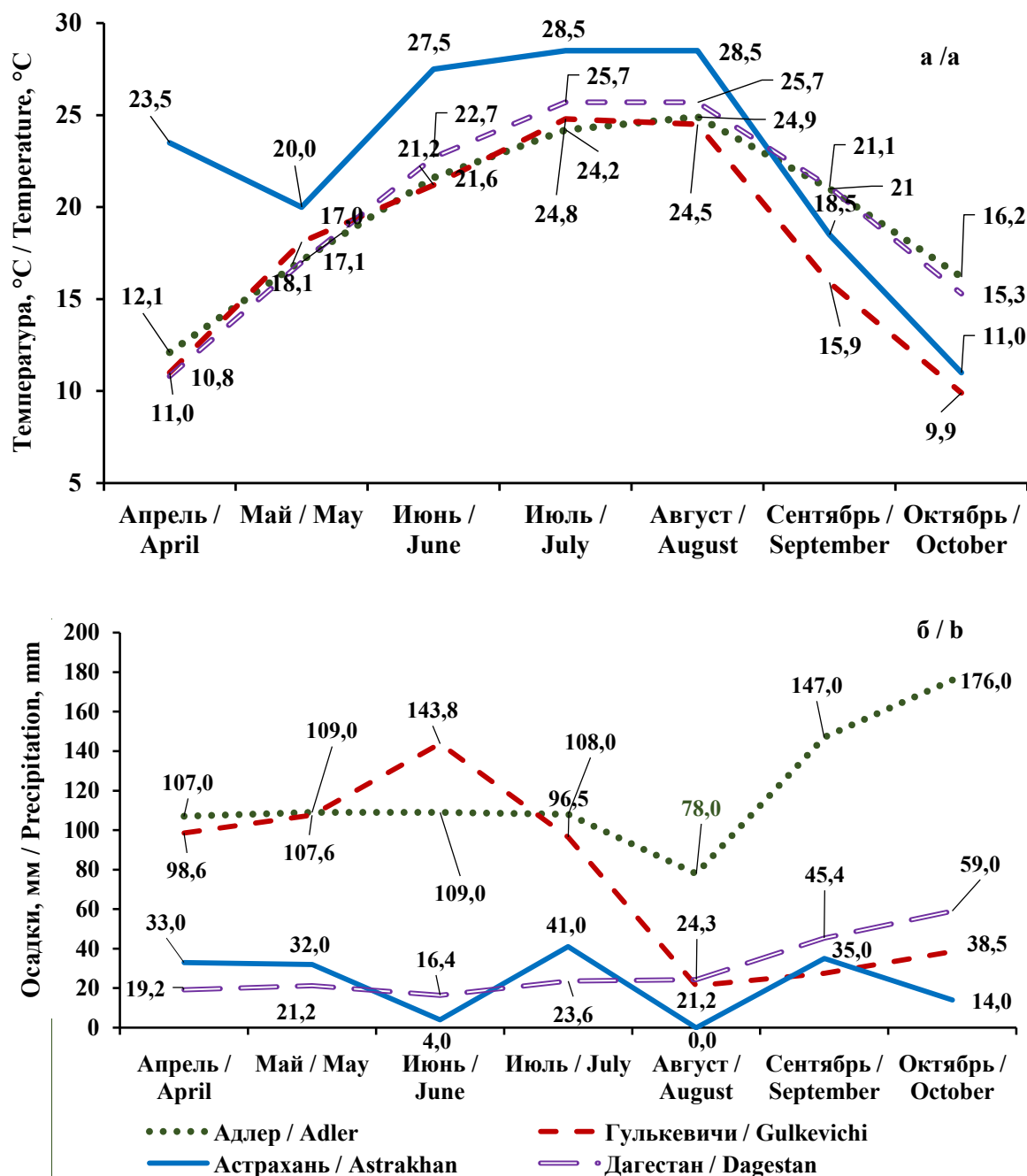
Рис. Гидротермические условия вегетации растений в регионах изучения (2018 г.): а – средне-месячная температура воздуха, °С; б – среднеемесячное количество осадков, мм
